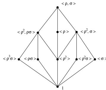
Figura 3.2: diagramma dei sottogruppi di D_8
